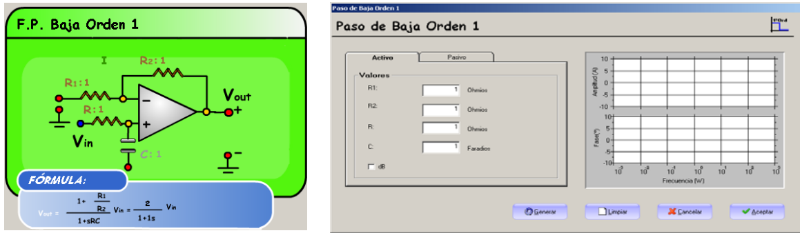
Figura 6: Filtro paso de baja de orden 1: Esquema, función de transferencia y captura de especificaciones.
